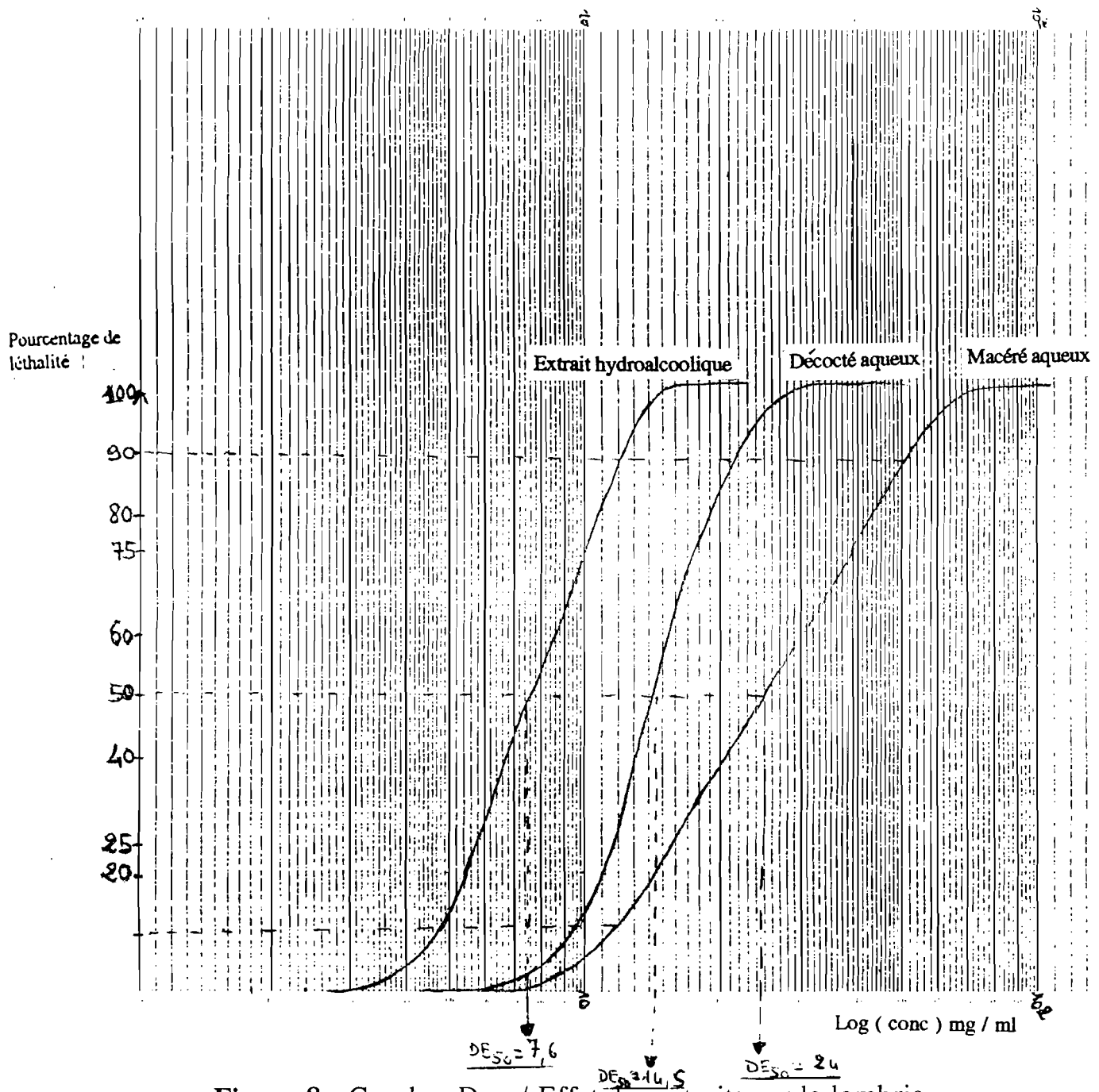
Figure 8 : Courbes Dose/ Effet des extraits sur le lombric
