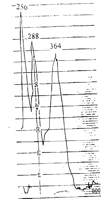
a : rutoside non complexé
