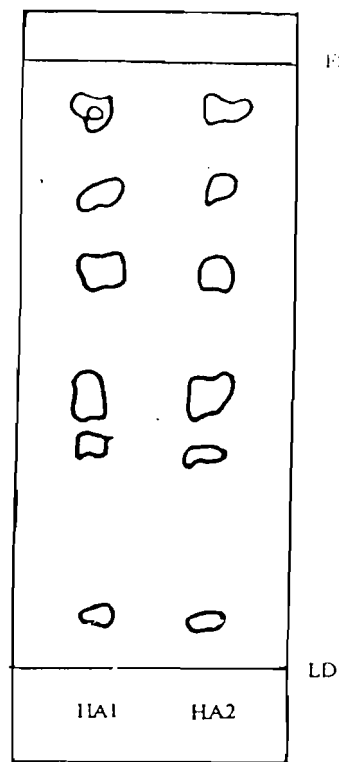
Chromatogramme 2 : CCM dans le solvant S1
