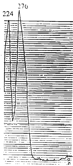
e : acide tannique non complexé
