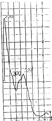
b : échantillon non complexé
