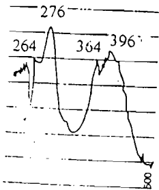
c : rutoside complexé
